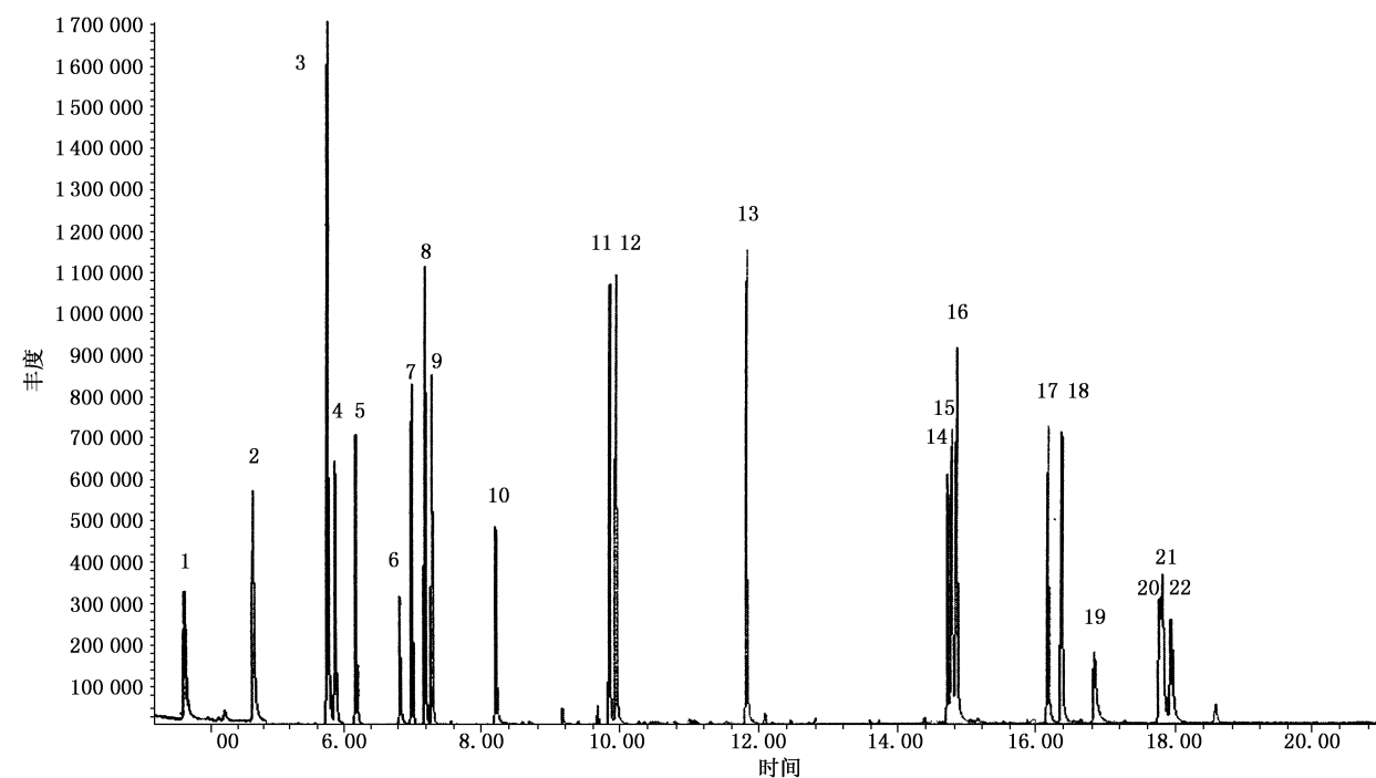
附录 C (资料性附录) 致癌芳香胺标准物色谱图
